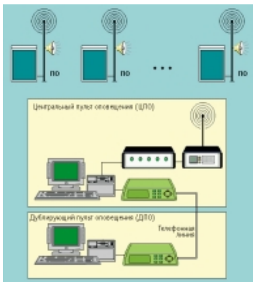
Рис. 1. Архитектура системы оповещения ПО — пост оповещения
